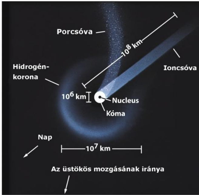
Az üstökösök főbb részei.
