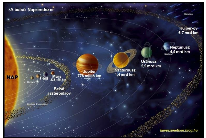
A belső Naprendszer
